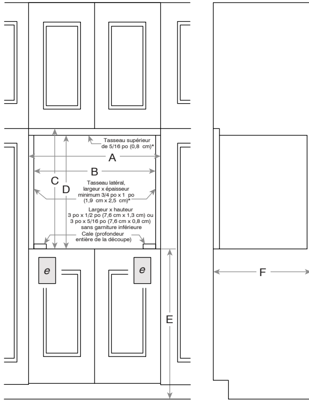
VUE AVANT
