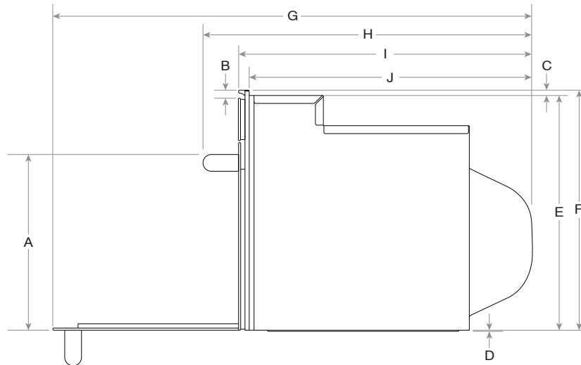
VUE LATÉRALE
