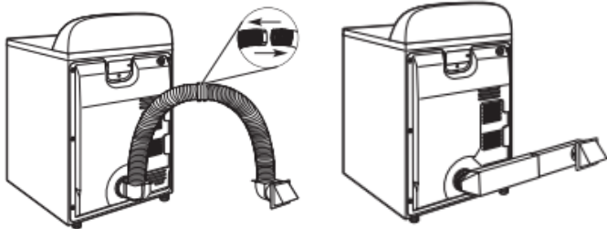
Installation au-dessus de la sècheuse Installation en périscopie (également offerte avec un coude décalé)
