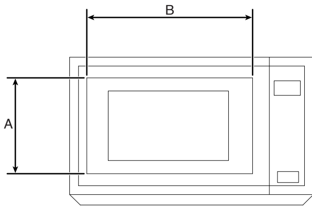
VUE AVANT INTÉRIÈRE DE LA CAVITÉ
